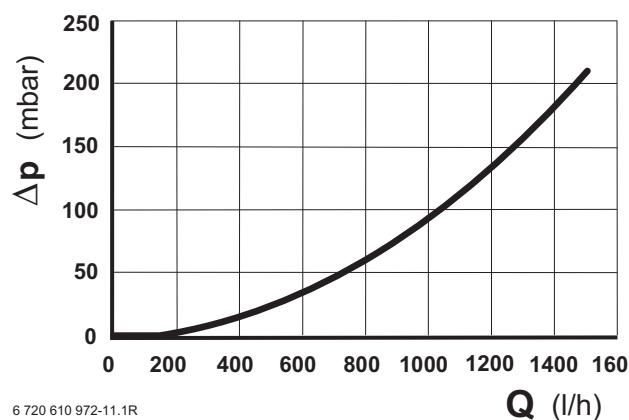
Fig. 11 Perdite di carico per apparecchi di tipo KBR
