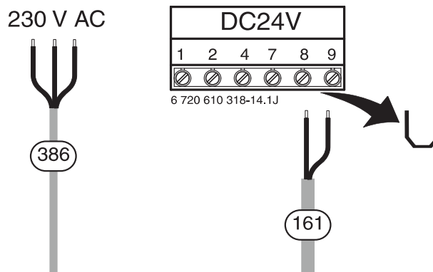
Fig. 20 Eliminare il collegamento con la Bosch Heatronic – ponticello 8-9!
