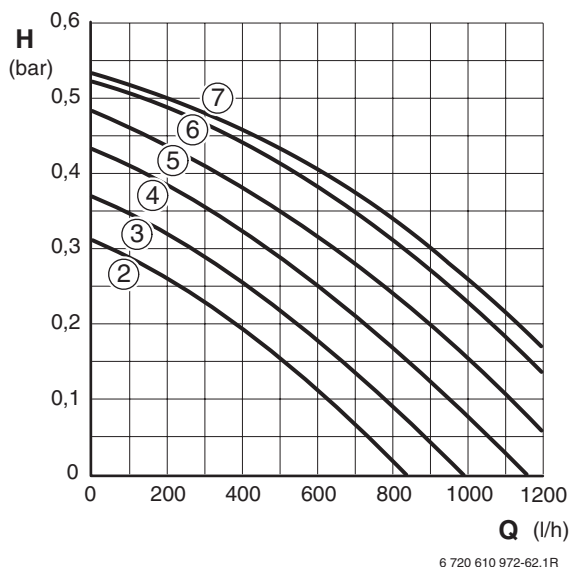
Fig. 64 Curve caratteristiche
